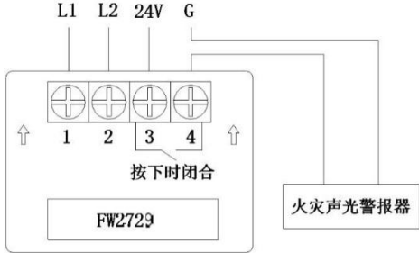
图 4-2 消火栓按钮 SLC 回路接线
