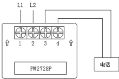
图 4-1 手动报警按钮 SLC 回路接线
