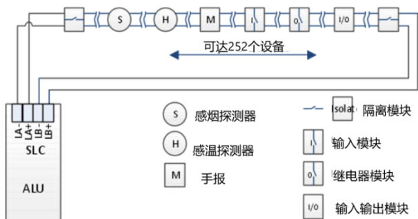
图 3 SLC 回路 Class A 接线
