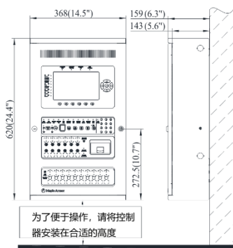
图 2-1 FW2105C 壁挂表面安装
