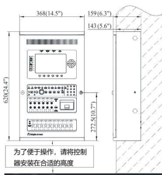
图 2-2 FW2105C 壁挂内嵌安装
