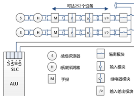
图 4 SLC 回路 Class B 接线
